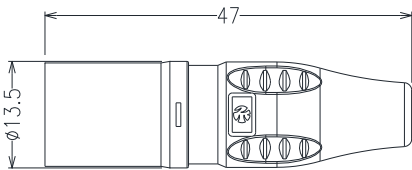
公连接器 Male Connector
